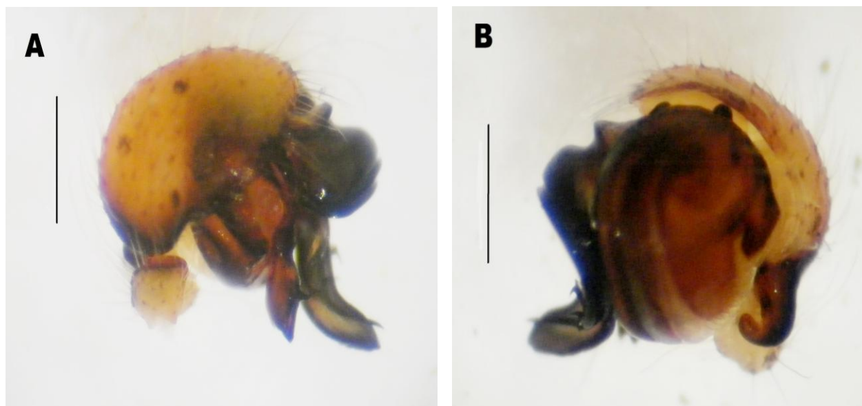
Figura 3. Palpo izquierdo del macho de A. argentata . A. Vista prolatral; B. Vista retrolateral. Escala: 0, 5 mm.
