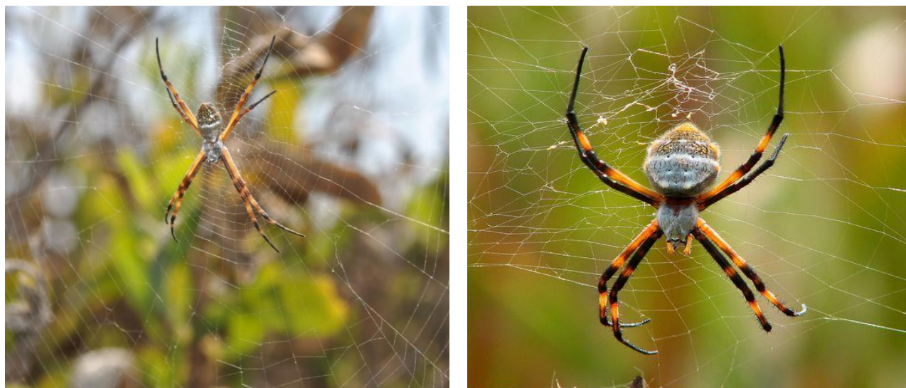
Figura 1. Habitus de Argiope argentata , Río Lluta. Izquierda: Posición clásica en forma de cruz; Derecha; Imagen dorsal ampliada de la especie.
